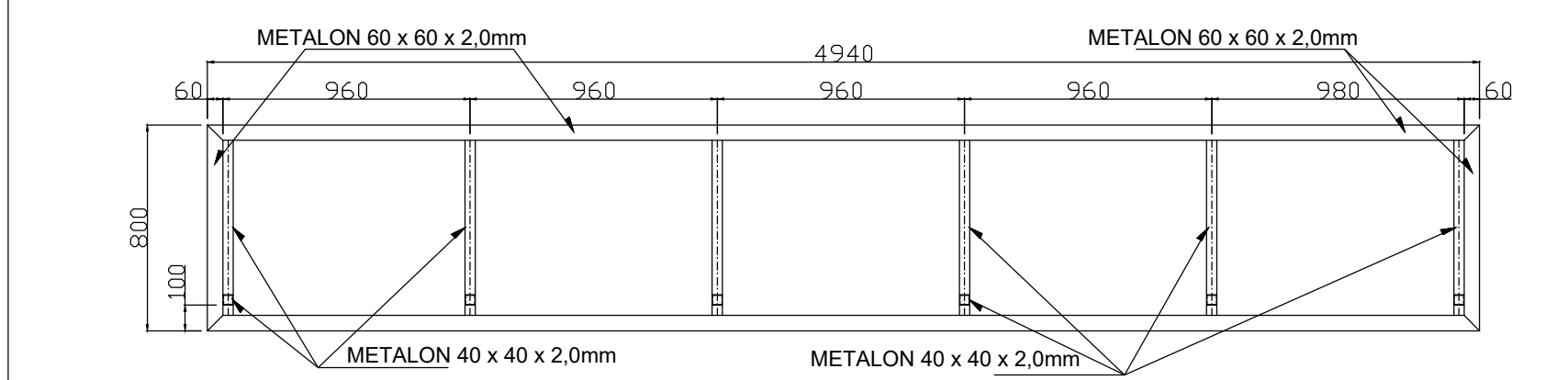
VISTA SUPERIOR
