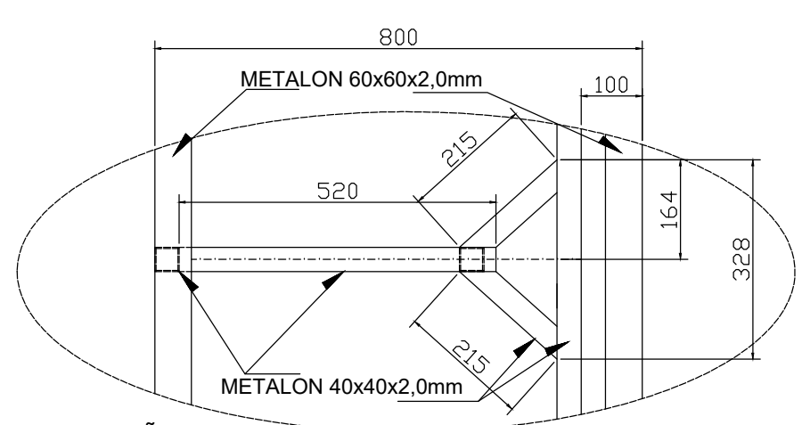
SEÇÃO BB
