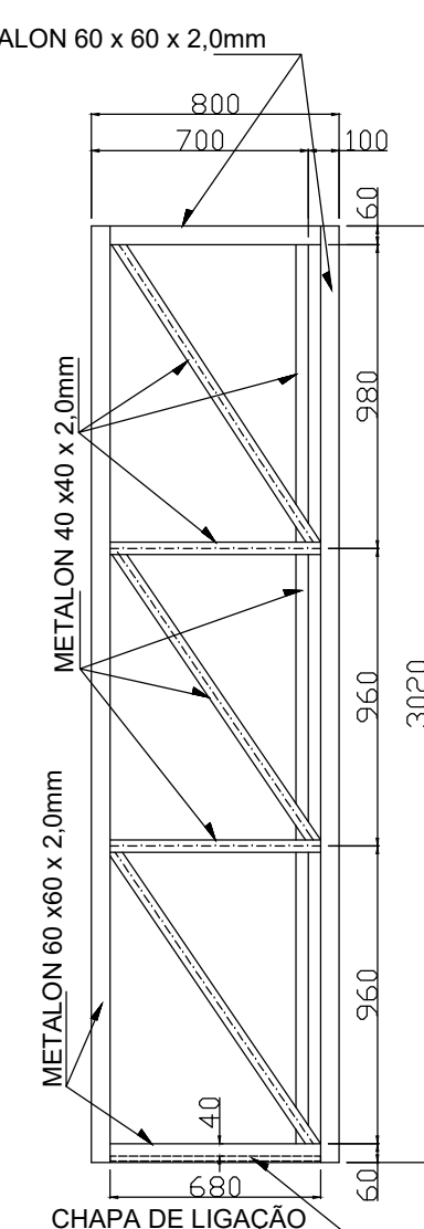
VISTA LATERAL
